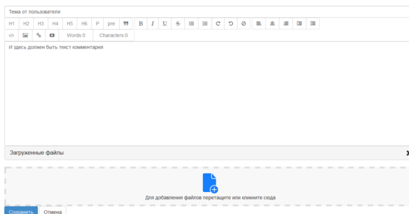
Рисунок 13 – Редактирование комментария
